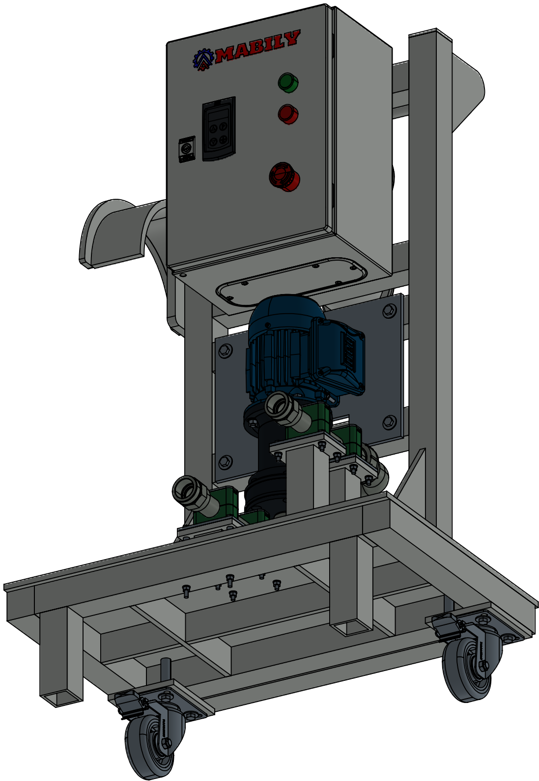
PERSPECTIVA INFERIOR - 1:5,88
