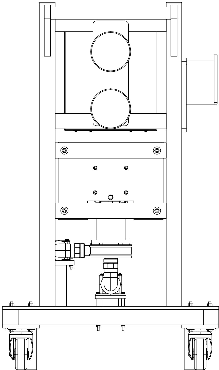
VISTA TRASEIRA
