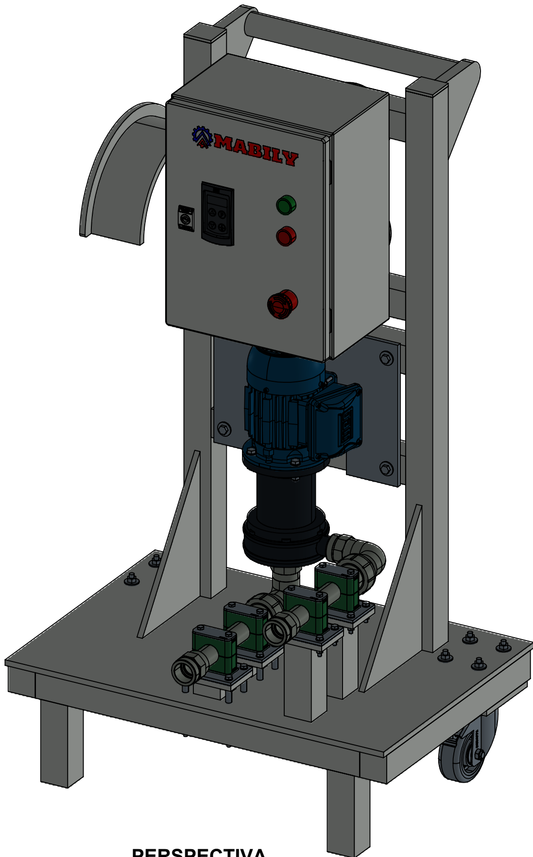
PERSPECTIVA
