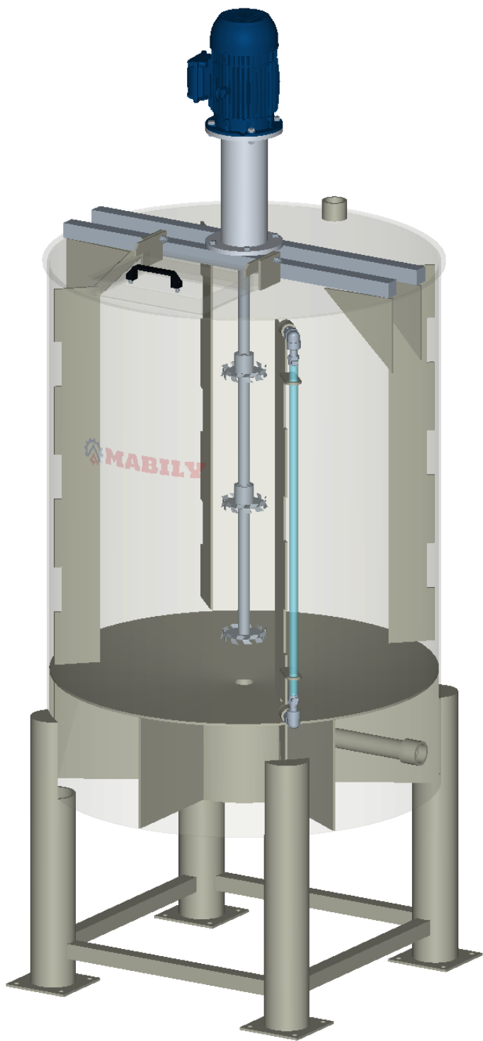
VISTA TRANSPARENTE
