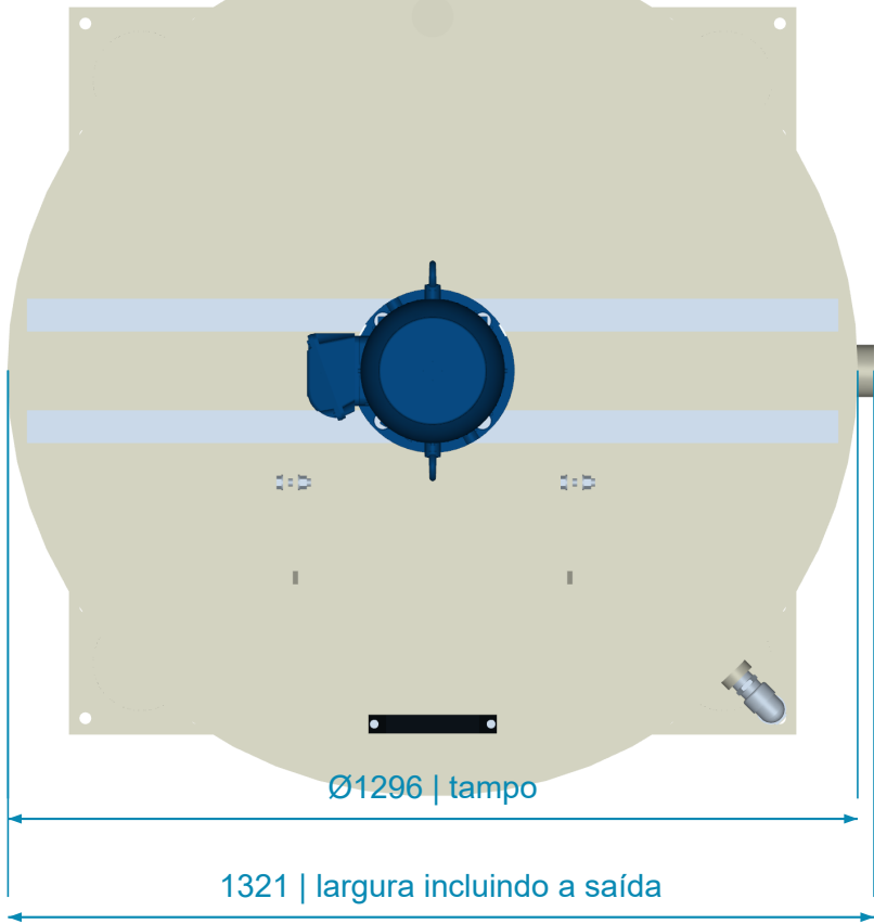
VISTA SUPERIOR
