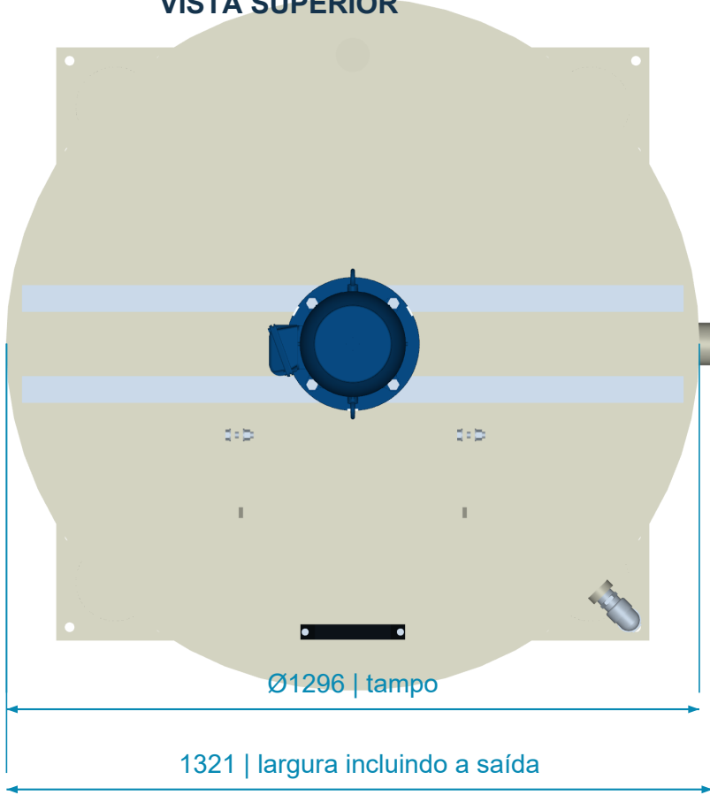
VISTA SUPERIOR
