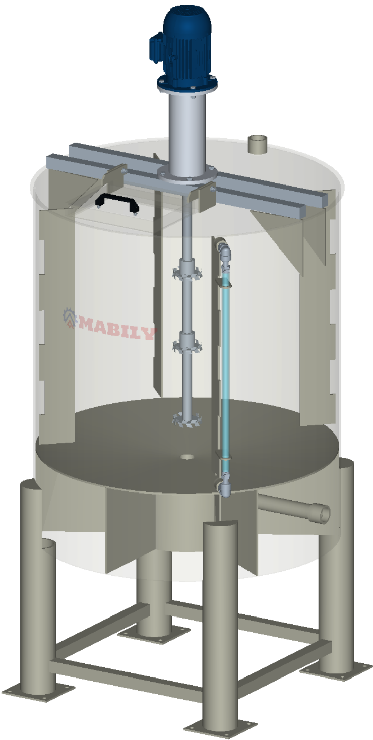
VISTA TRANSPARENTE
