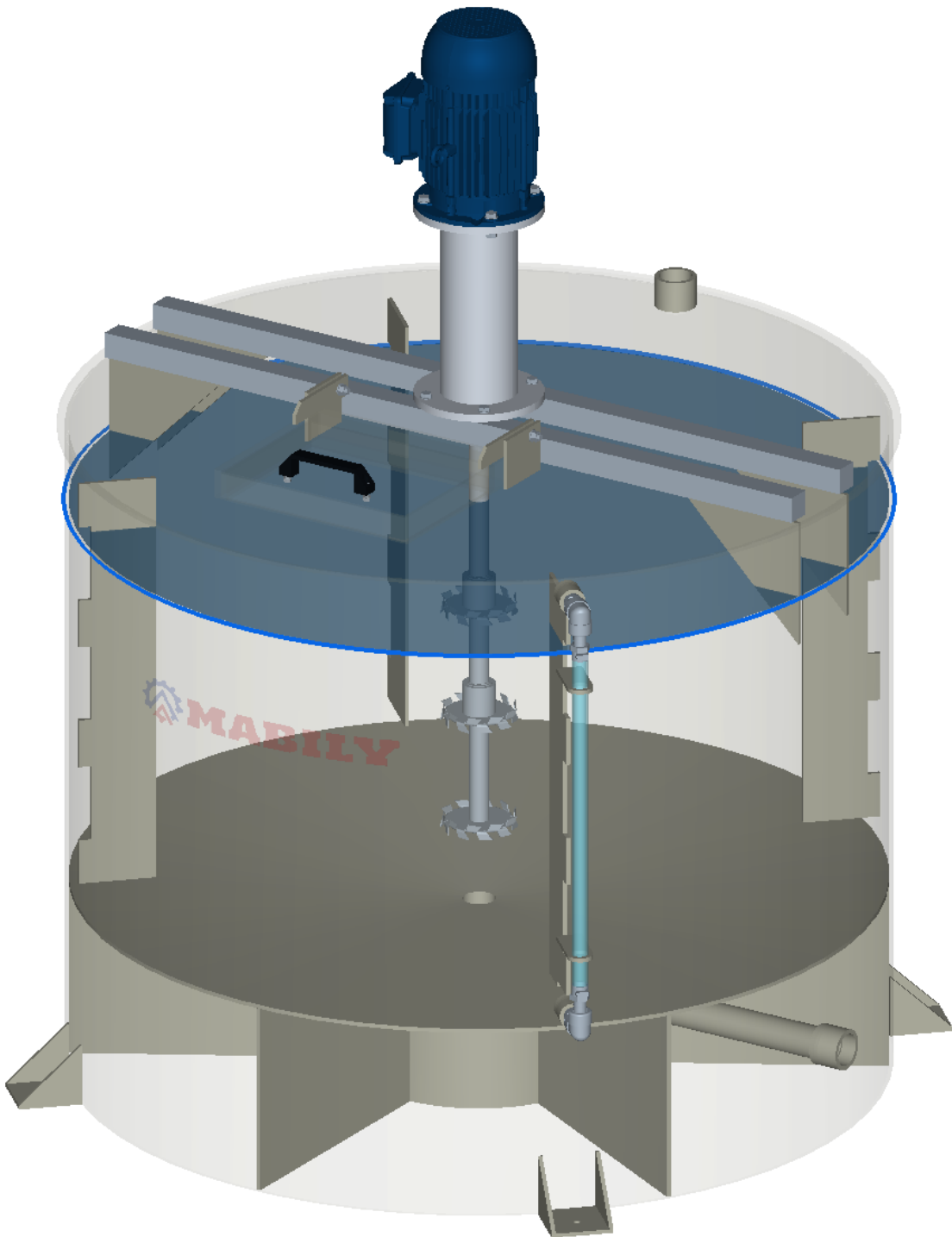
INTERIOR E LINHA D'ÁGUA
